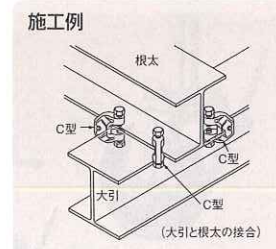
施工例 (大引と根太の接合)
