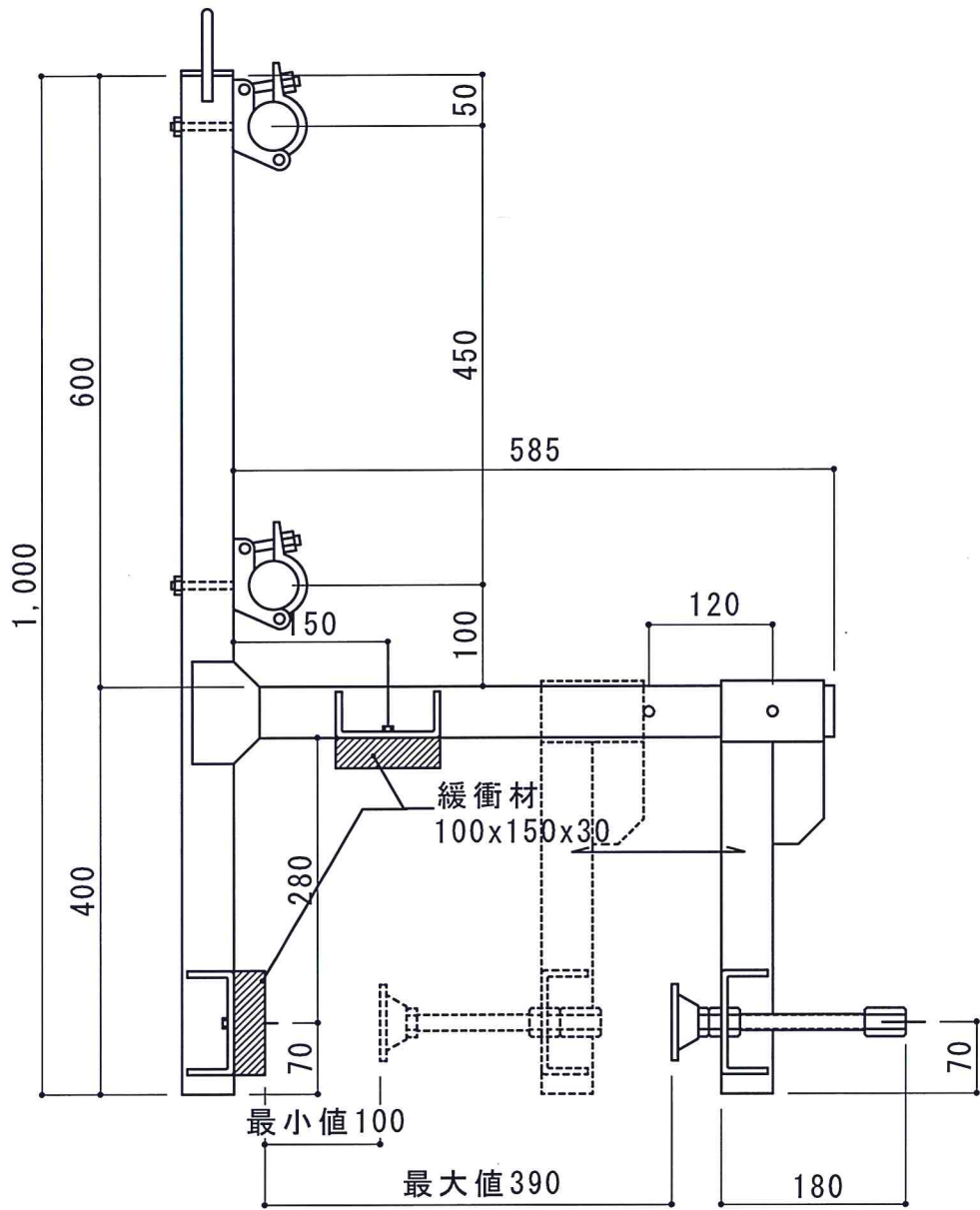
正面図
