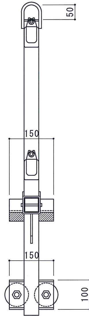
側面図
