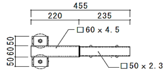
上面図
